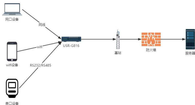
图 4 应用示意图
